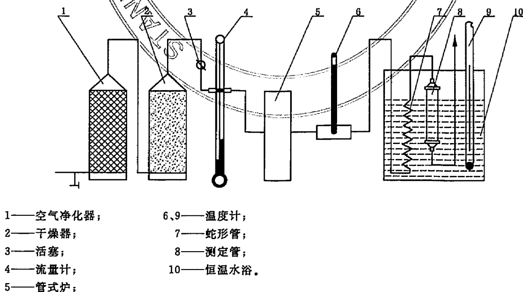
图 1 脱附率试验装置示意图
